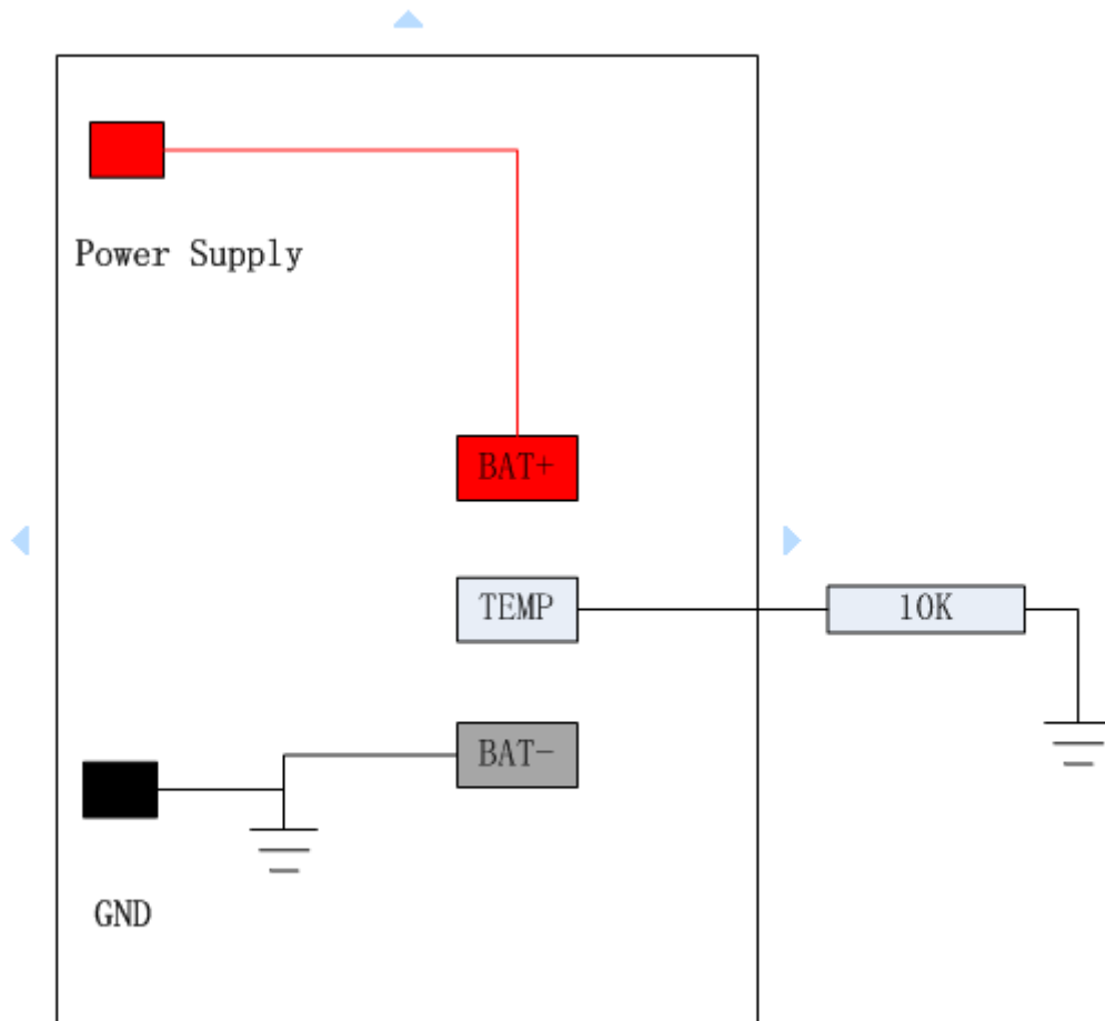
图 4.2 NTC 夹具接线方法
